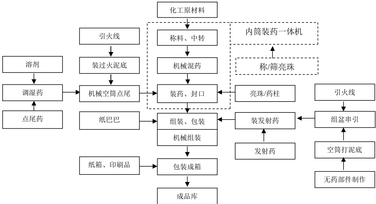
图 2-1：组合烟花类生产工艺流程图
